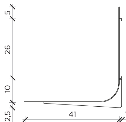
LATO | SIDE
