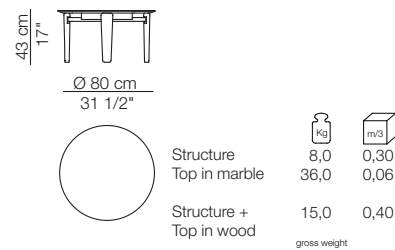
Tavolino Ø 80 H.43 cm Small table Ø 80 H.43 cm
