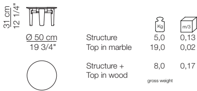
Tavolino Ø 50 H.31 cm Small table Ø 50 H.31 cm
