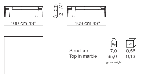
Tavolino 109 x 109 H.31 cm Small table 109 x 109 H.31 cm
