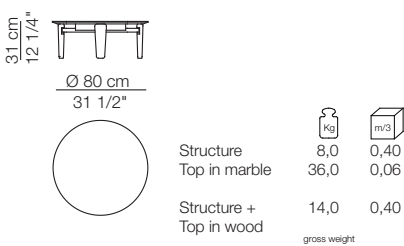
Tavolino Ø 80 H.31 cm Small table Ø 80 H.31 cm
